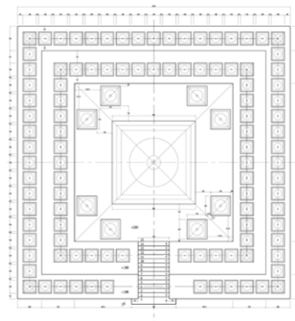
敦珠佛母舍利塔平面圖
